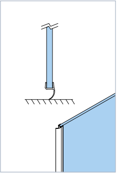
CIERRE SOLAPE DE SERIE
