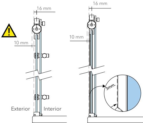
Opción con soportes a pared
