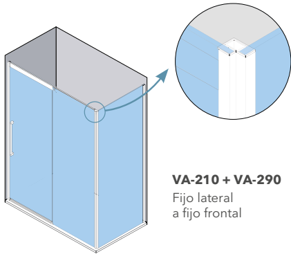
VA-210 + VA-290 Fijo lateral a hoja corredera
