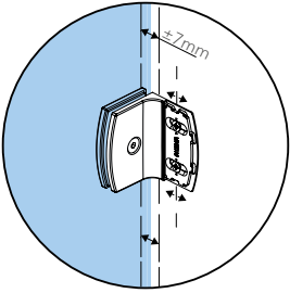
Fija pared-vidrio 90°
