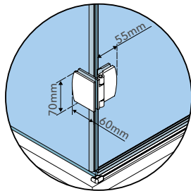
Bisagra vidrio-vidrio 90°
