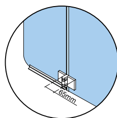
Detalle interior: Bisagra Belus apertura 180° (Posición cerrada)
