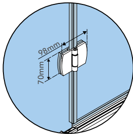
Bisagra vidrio-vidrio 180°
