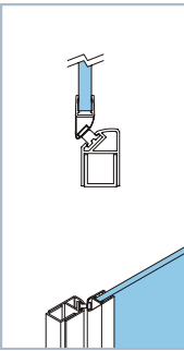
REFERENCIADO: Perfil con cierre magnético. Apertura exterior.
