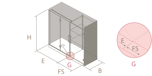
Detalle puerta abierta
