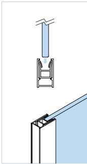
Perfil con cierre junquillo.
