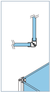
Cierre magnético. Apertura interior y exterior.
